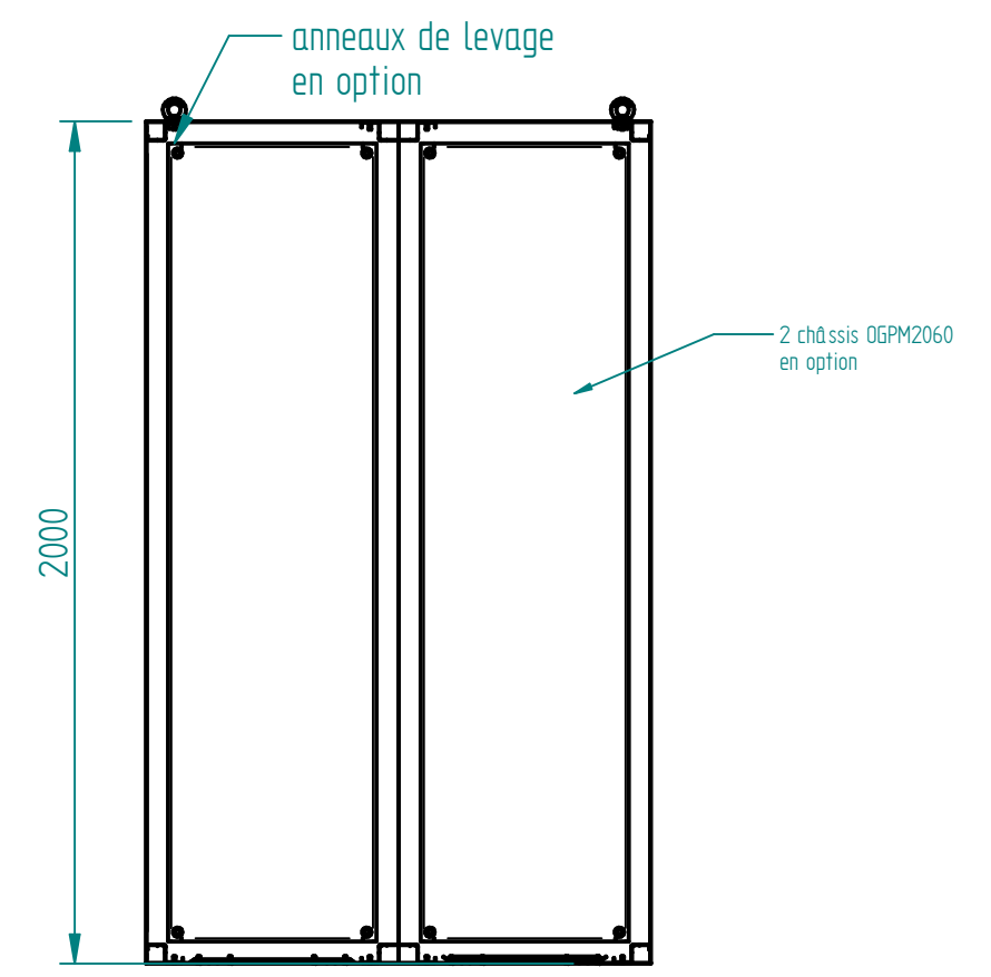
COUPE B-B
